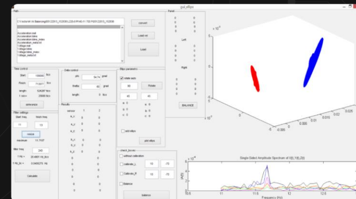
Траекторный вид ротора после балансировки
