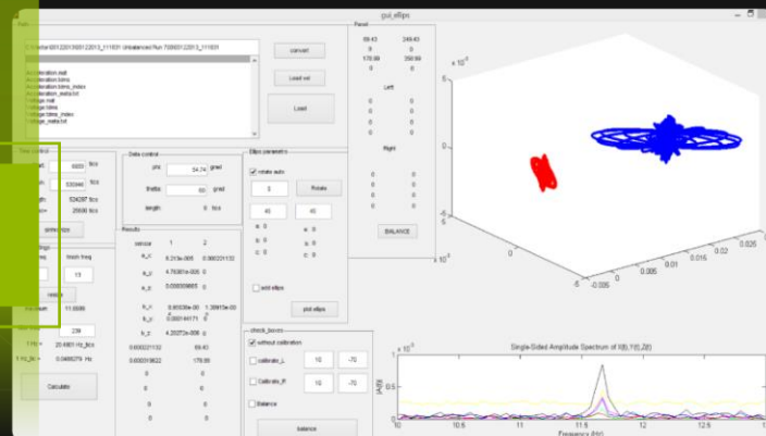
Траекторный вид ротора до балансировки
