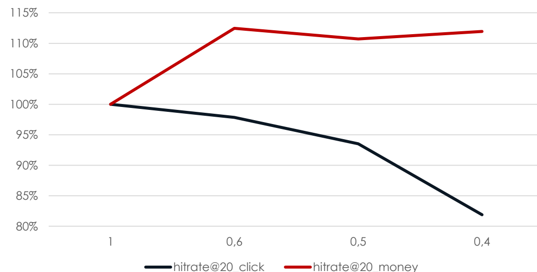
HITRATE при снижении веса ТДД
